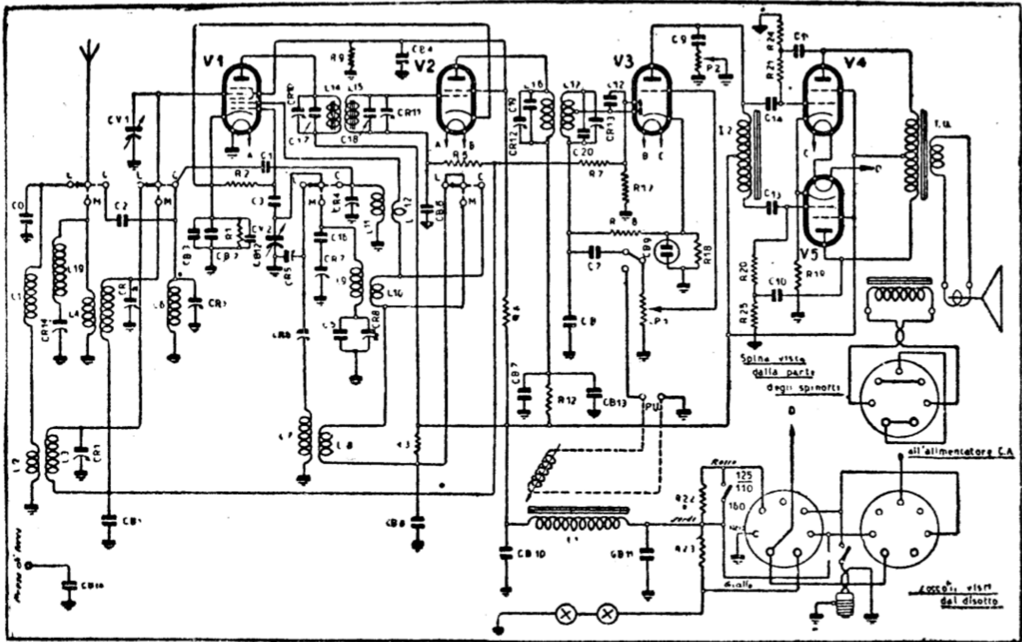
RADIO SAFAR. — Mod. 634 C. C. — Per reti a corrente continua. — MF: 470 kHz. Produzione 1938.
